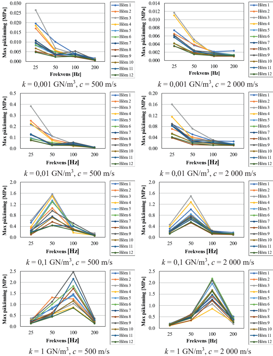
Figur 3.15 Maximala påkänningar i Vägg 2 (lättbetongvägg) vid varierende värde på markstyvhet k , lastfrekvens f och våghastighet c . Maximum stresses in Wall 2 (lightweight concrete wall) at varying values of ground stiffness k , load frequency f and wave speed c .
