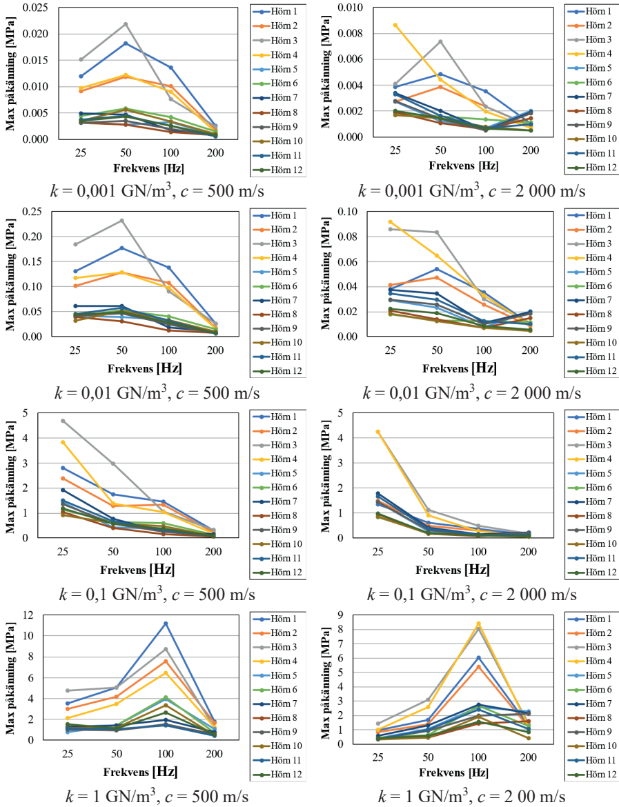
Figur 3.13 Maximala påkänningar i Vägg 2 (betongvägg) vid varierande värde på markstyvhets k , lastfrekvens f och våghastighet c . Maximum stresses in Wall 2 (concrete wall) at varying values of ground stiffness k , load frequency f and wave speed c .
