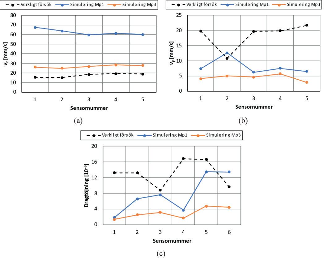
Figur 4.16 Jämförelse mellan försök och simuleringar för Salva 2.2: (a) maximal vertikal hastighet, (b) maximal horisontell hastighet och (c) maximal dragtöjning. Comparison between experiments and simulations for Blast round 2.2: (a) maximum vertical velocity, (b) maximum horizontal velocity, (c) maximum tensile strain.
