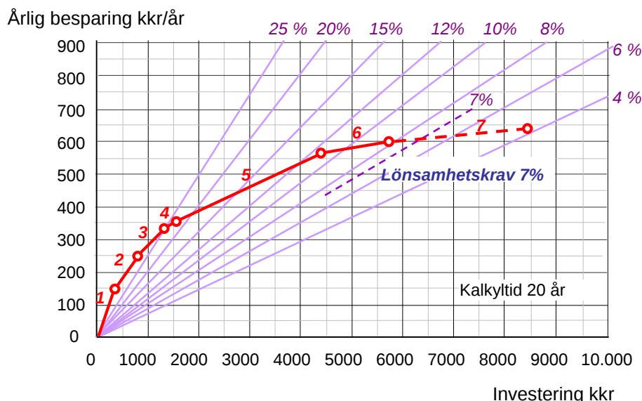
Figur 2.14 Åtgärdernas lönsamhet presenterad i ett internräntediagram och bildning av åtgärdspaket. Procentsatserna anger internräntan. Beställarens lönsamhetskrav är 7 %. Notera att alla åtgärder i det visade exemplet har samma kalkyltid, 20 år.
