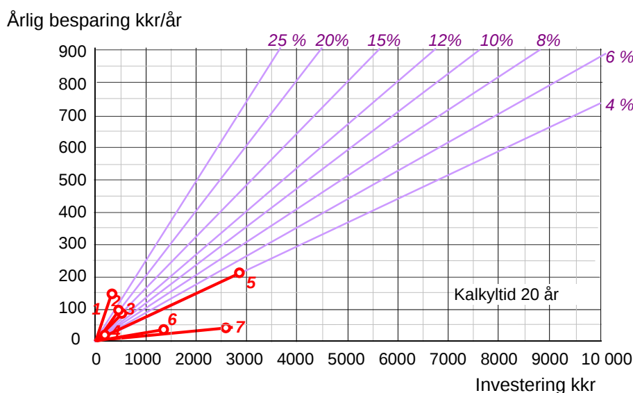
Figur 2.13 Åtgärdernas lönsamhet presenterad i ett internräntediagram. Procentsatserna anger internräntan. Råda punkter med linjer till origo representerar olika åtgärder. Diagrammet gäller för kalkyltiden 20 år.
