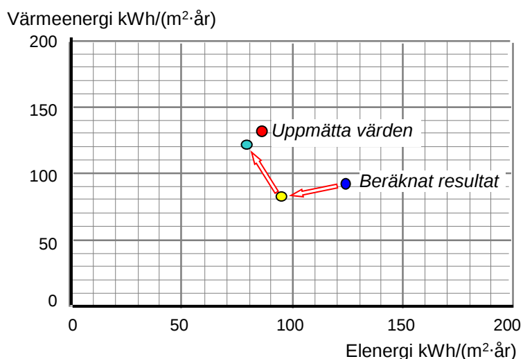
Figur 6.4 Jämförelse av resultaten av energiberäkningar med uppmätt energianvändning efter justering av osäkra indata.
