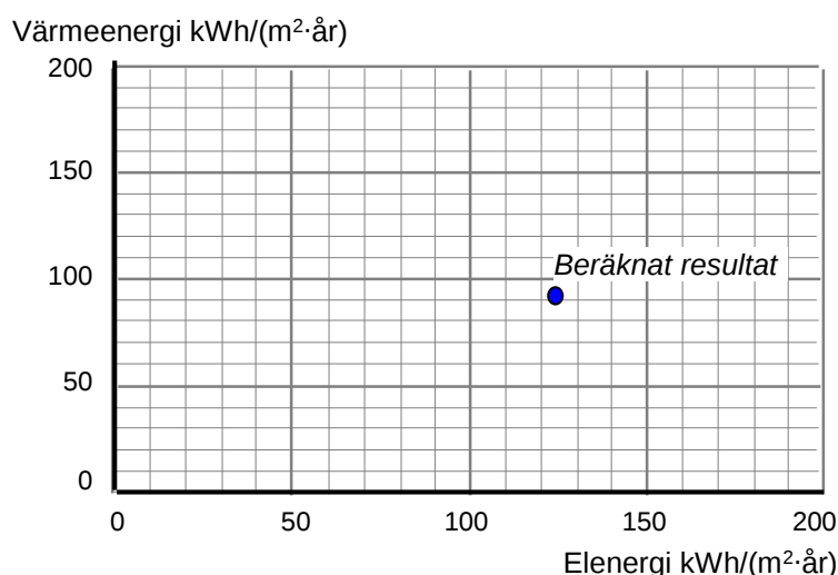
Figur 6.2 Resultaten av första beräkning i energiberäkningsprocessen: energi-användning för värme och el.
