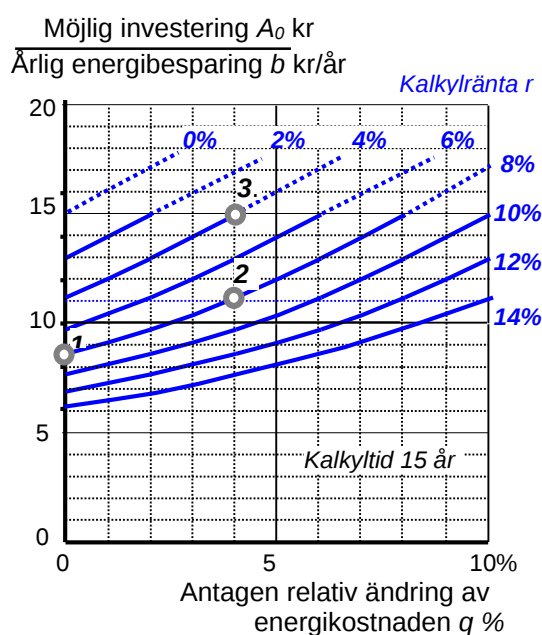
Figur 2.3 Inverkan på en lönsamhetsbedömning av valet av kalkylränta och antagande om framtida energiprishöjning.
