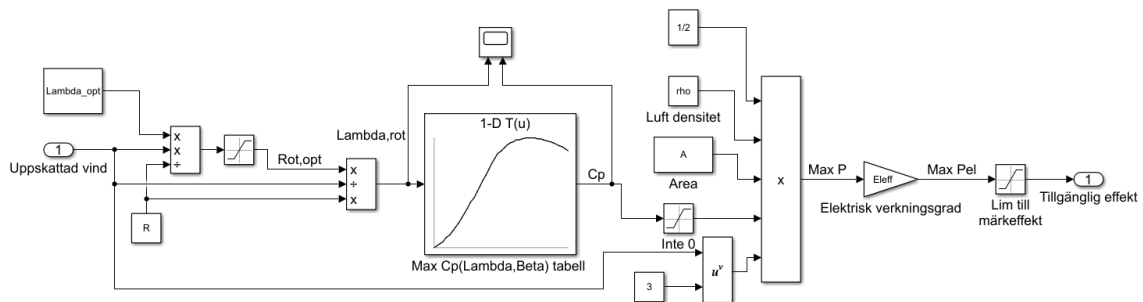
Figur 6: Blockschema över processen för att uppskatta maximalt tillgänglig effekt från en vindhastighet
