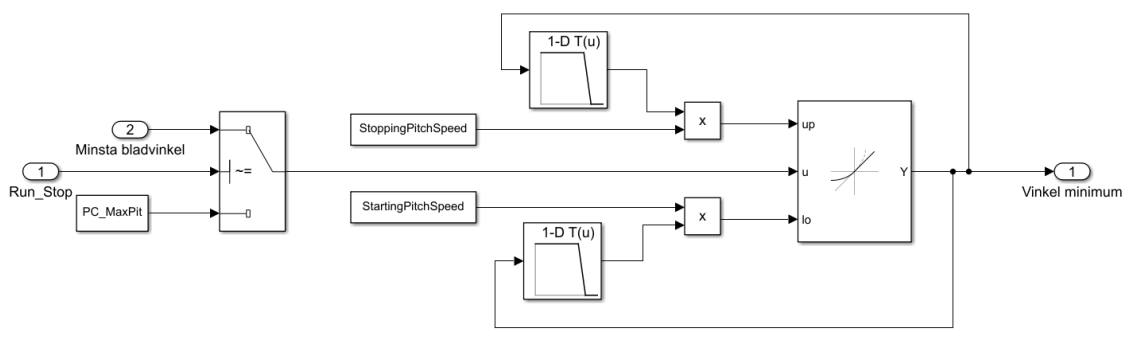
Figur 16: Inre schema för blocket "Start-stop"
