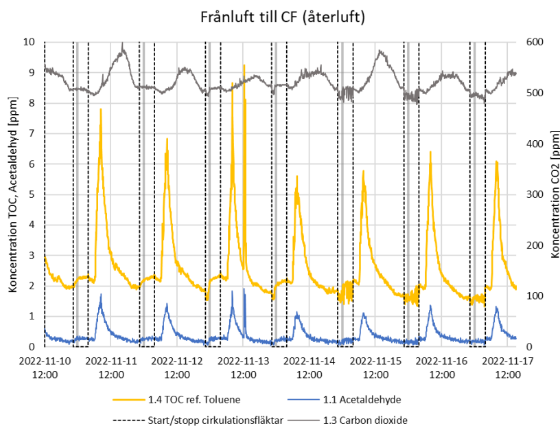
Figur 15 Koncentration av TVOC (ref. Toluene) och totala aldehyder (ref. Acetaldehyd) i frånluft till cirkulationsfläktar (återluft), butik B.
