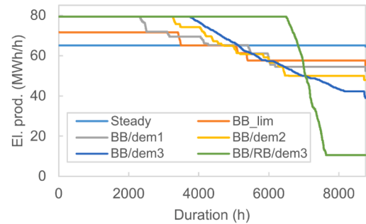
(d) Cond. turbine electricity production.
