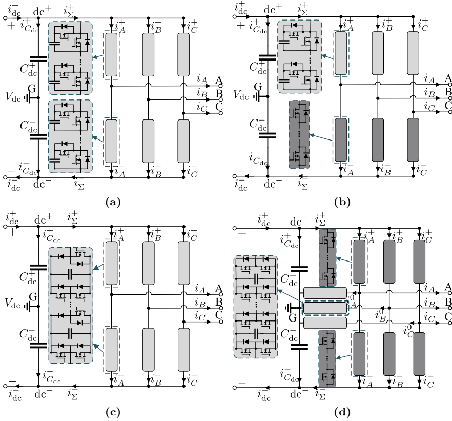
Figure 2.4: Multilevel converters (a) MMC. (b) TAC. (c) MTAC. (d) CTB converter.
