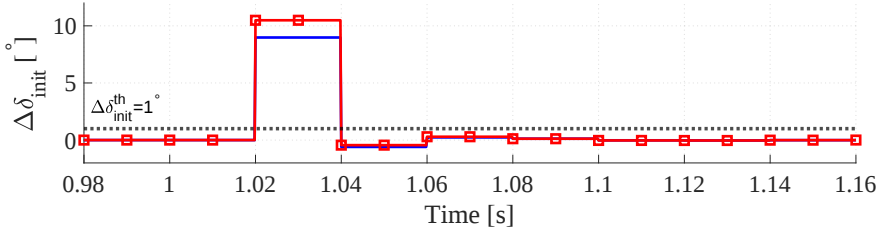
(d) Cycle-to-cycle load angle jump
