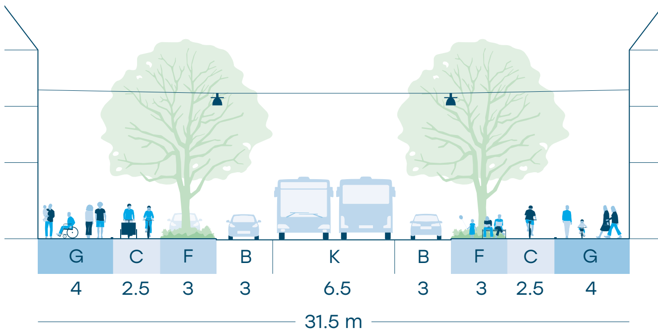
Sektion med minimimått.
