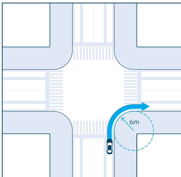
Körfälts standardradie i gatukorsningar i huvudgatunätet, 6 meter.
