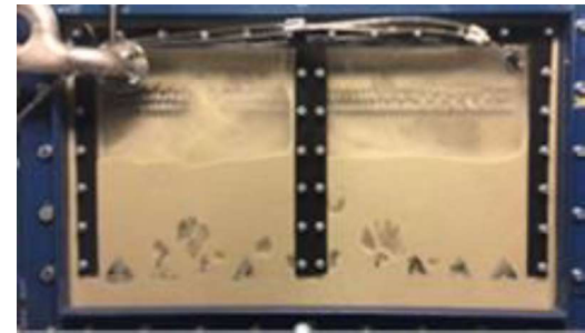
(d) 0.6 m/s, V_{sv} \sim 30\% , VD Mode 1B with Internal baffles, AD 198
