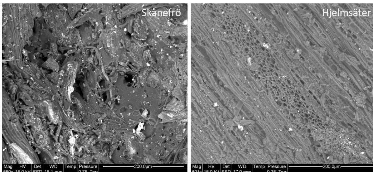
Figur 2. Svepelektronmikroskopi (SEM) av biokol från Skånefrö och Hjelmsäter.
