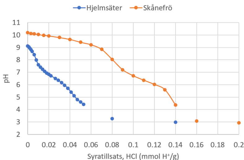
Figur 3. Titreringskurvor för biokolen. De separata punkterna visar mätningar som gjordes vid ett senare tillfälle för att visa den syratillförsel som krävdes för att sänka pH till 3.
