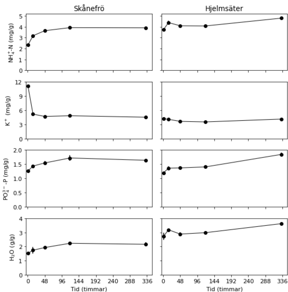
Figur 4. Mängd ammonium (NH 4 + ), kalium (K + ), fosfat (PO 4 3- ) och vatten (H 2 O) bundet till biokol från Skånefrö (vänster) och Hjelmsäter (höger) efter olika kontakttider. Medelvärde från duplikat visas. Felstaplar visar minimum- och maximumvärden.
