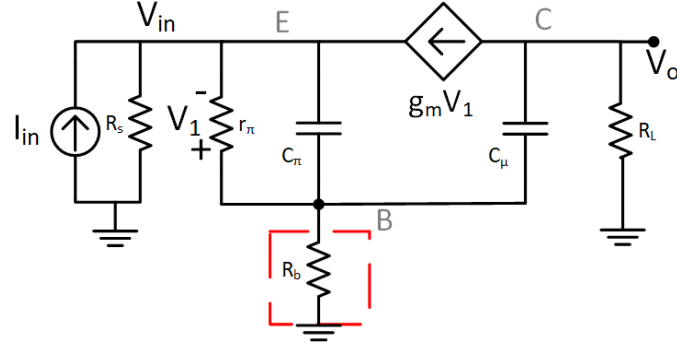
(d) CB small signal high frequency circuit.
