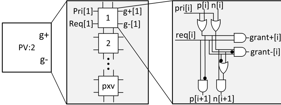
(b) PV:2 output arbiter.
