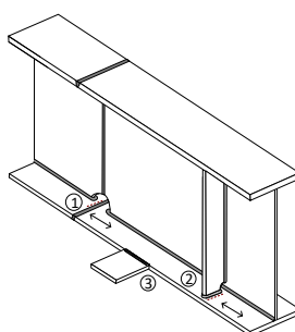
Figur 1. Illustration av de utvalda kritiska detaljerna som bestämmer utmattningslivet för en brobalk.
