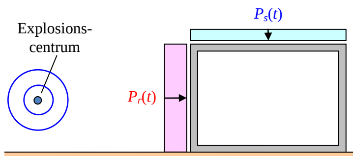
Figur 3.4 Utvändig explosion mot byggnad. Vid belastning med ett reflekterat tryck P_r mot den närmaste fasadväggen så kommer det samtidigt verka ett oreflektat tryck P_s mot taket. Lasten mot taket kommer i sin tur, via sin stödreaktion, ge upphov till en normalkraft mot väggen.
