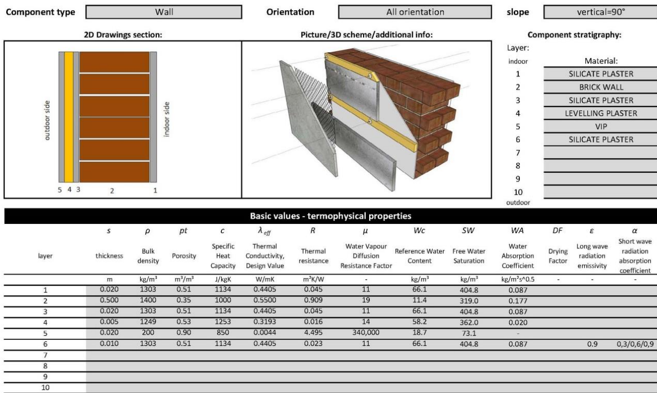
Figure Erreur ! Il n'y a pas de texte répondant à ce style dans ce document.-1. Summary data-sheet of the analysed wall.
