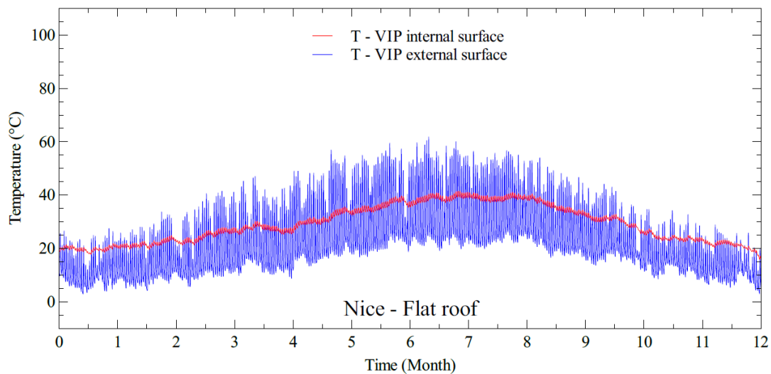
Figure Erreur ! Il n'y a pas de texte répondant à ce style dans ce document. -45 : Temperatures evolution over one year, at the VIPs' internal and external surfaces, for flat roof in Nice.
