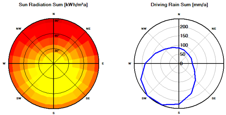
Figure Erreur ! Il n'y a pas de texte répondant à ce style dans ce document.-10.-: Solar radiation (left), driving rain and mean wind speed (right).
