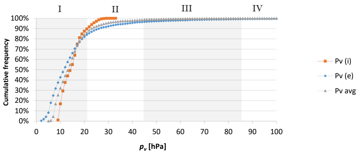
Figure Erreur ! Il n'y a pas de texte répondant à ce style dans ce document. -31. Vapour pressure cumulative functions for the south dark pitched roof, medium internal moisture load, VIP thickness 20 mm.
