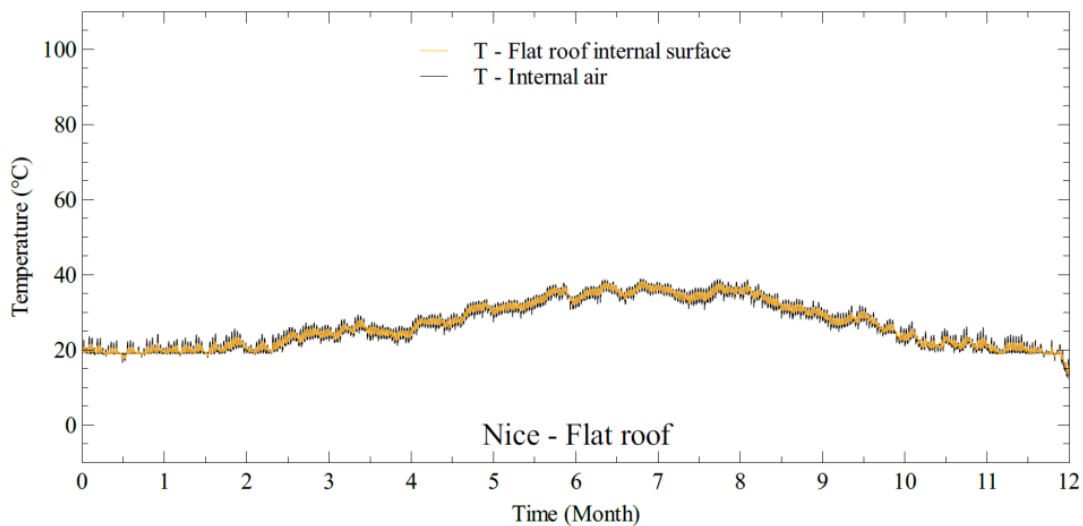
Figure Erreur ! Il n'y a pas de texte répondant à ce style dans ce document.-18. Yearly time profile of temperatures of internal air and at the internal wall surface.
