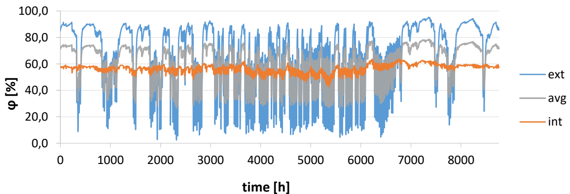
Figure Erreur ! Il n'y a pas de texte répondant à ce style dans ce document. -27. Yearly time profile of \phi s for the south dark pitched roof, medium internal moisture load, VIP thickness 20 mm.
