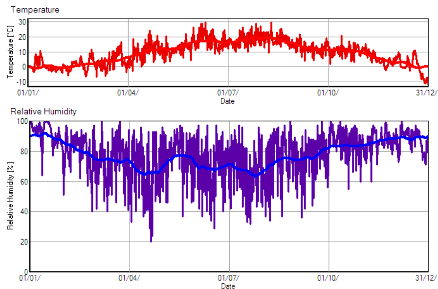
Figure Erreur ! Il n'y a pas de texte répondant à ce style dans ce document.-9. Outdoor temperature (upper), outdoor relative humidity (below).
