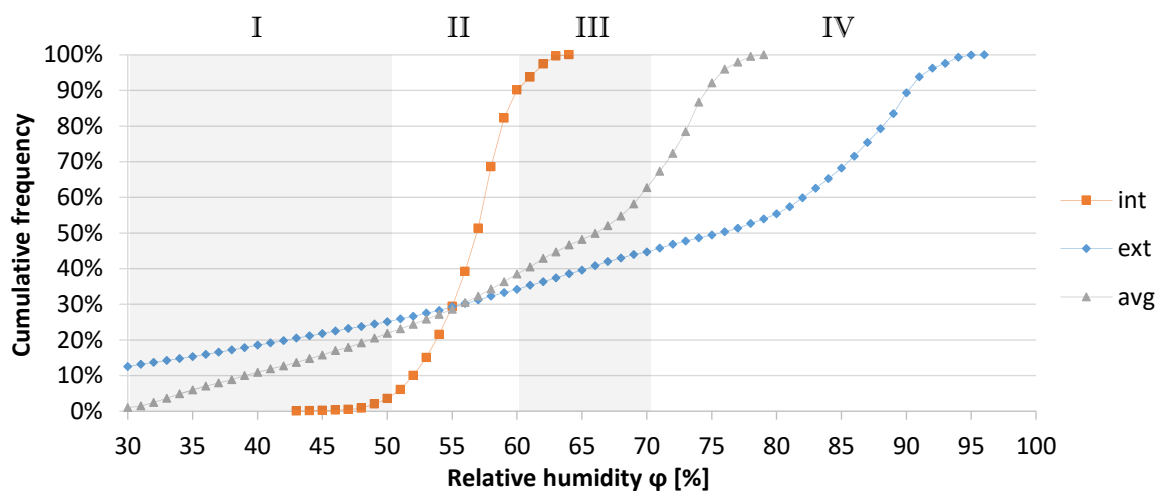
Figure Erreur ! Il n'y a pas de texte répondant à ce style dans ce document. -30. Relative humidity cumulative functions for the south dark pitched roof, medium internal moisture load, VIP thickness 20 mm.
