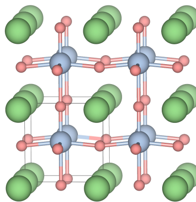
(d) The Tetragonal P4mm (99) crystal symmetry.
