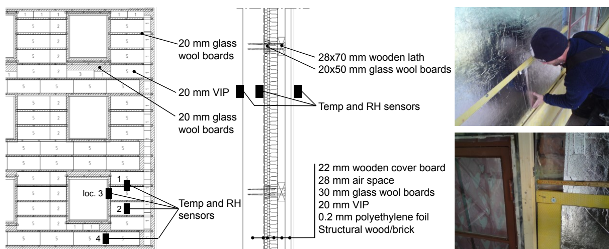
Figur 5: Vänster: Väggen efter tilläggsisolering med 20 mm VIP och 30 mm mineralullsskiva. Placering av sensorer för temperatur och relativ fuktighet markeras med de svarta rektanglarna; 1) bakom mineralull, 2) mitt bakom VIP, 3) vid fönsterkarm, 4) bakom anslutning mellan två VIP. Höger: Montering av VIP där mineralullen skapar en köldbrygga mellan panelerna och mellan paneler och fönster.
