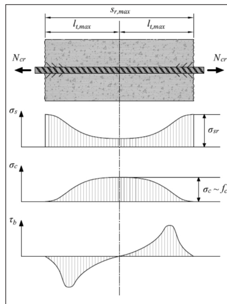
Figur 3: Fördelning av stål-, betong och vidhäftningspåkänningar i en armerad betongstav vid spricka.
