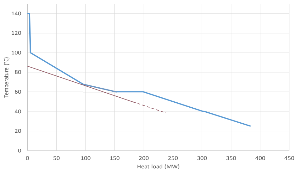
Figur 3. Praktiskt tillgänglig värme i Stenungsundsindustrierna enligt tidigare studier (blå linje), samt möjligt internt uppsamlingssystem (brun linje).
