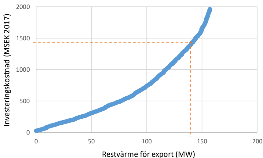
Figur 4. Kostnad för ett uppsamlingssystem av värmen samt fjärrvärmeväxlare (exklusive kostnader för inter användning). Exempelvis 1420 MSEK med 140 MW restvärme.
