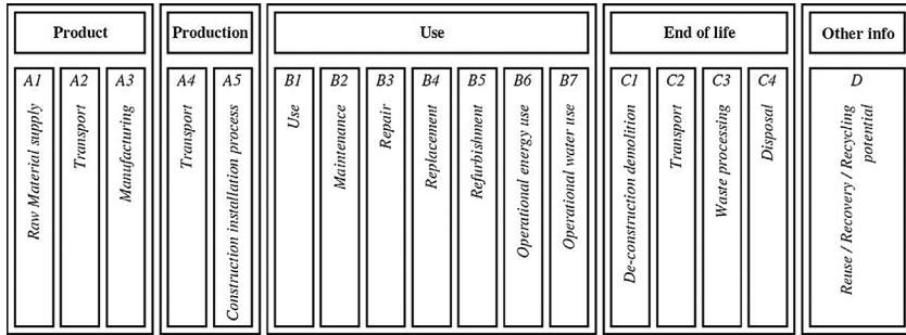
Fig. 1. Overview of the life cycle modules of a building (EN 15804).
