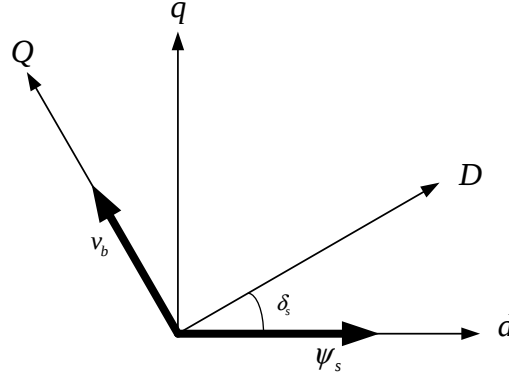
Fig. 2.12 Relation between dq and DQ frame.
